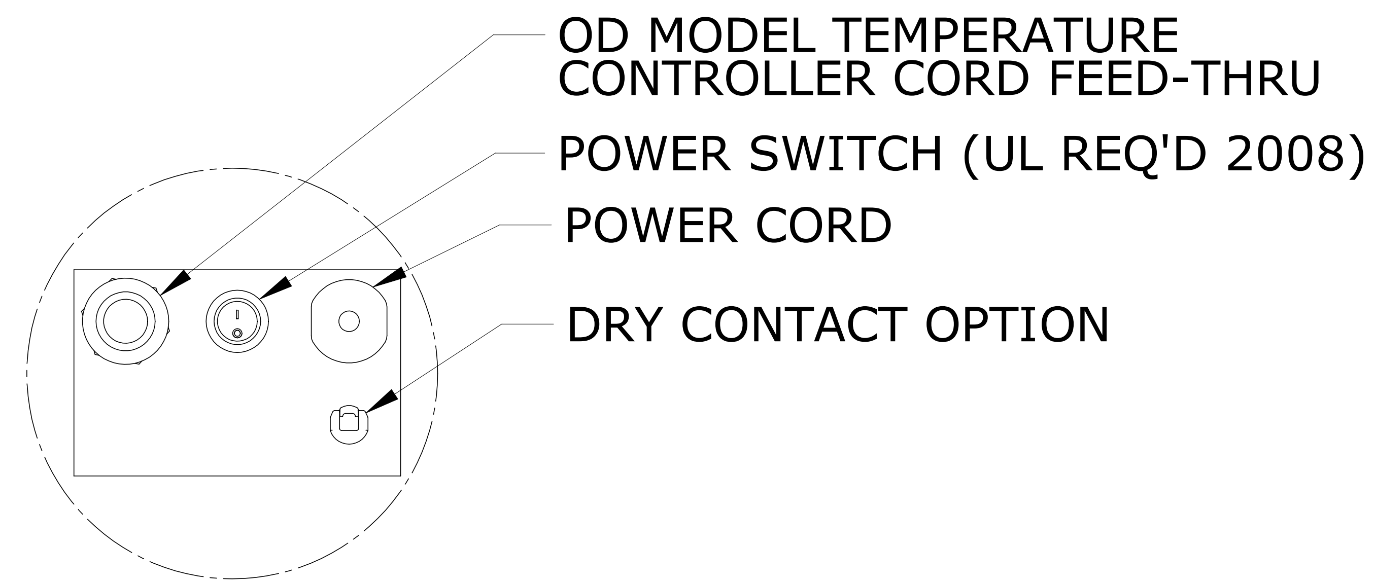
DETAIL A 2:1
