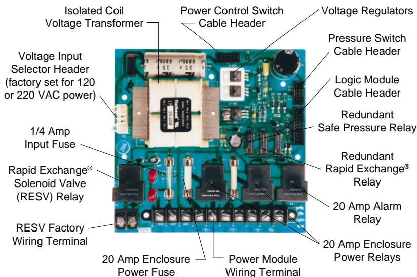
120/220 VAC EPCU Power Module
