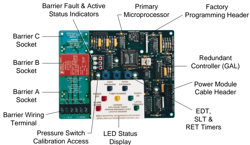
EPCU Logic Module
